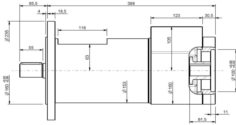
SEZIONE H-H
