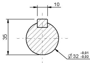
SEZIONE H-H
