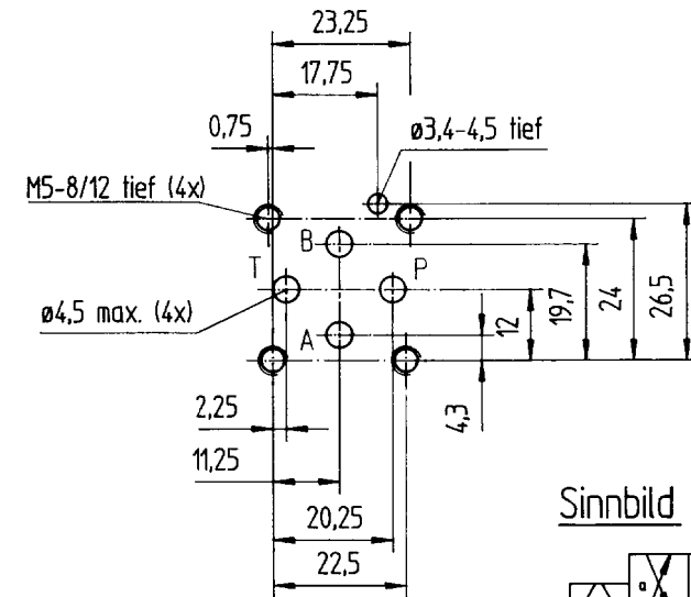
Anschlußbild
